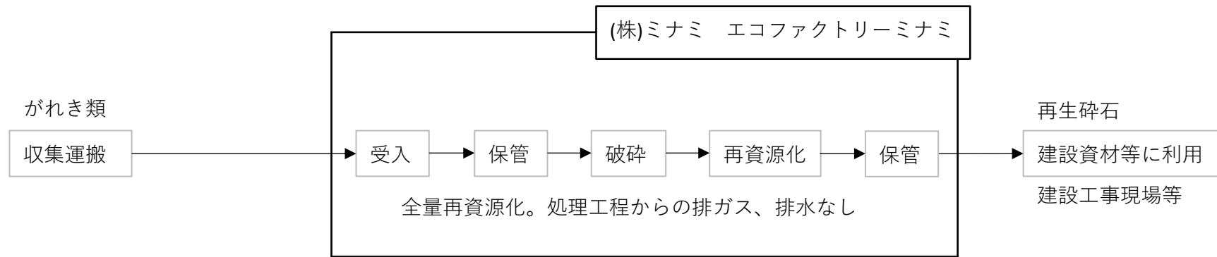
処理工程図
